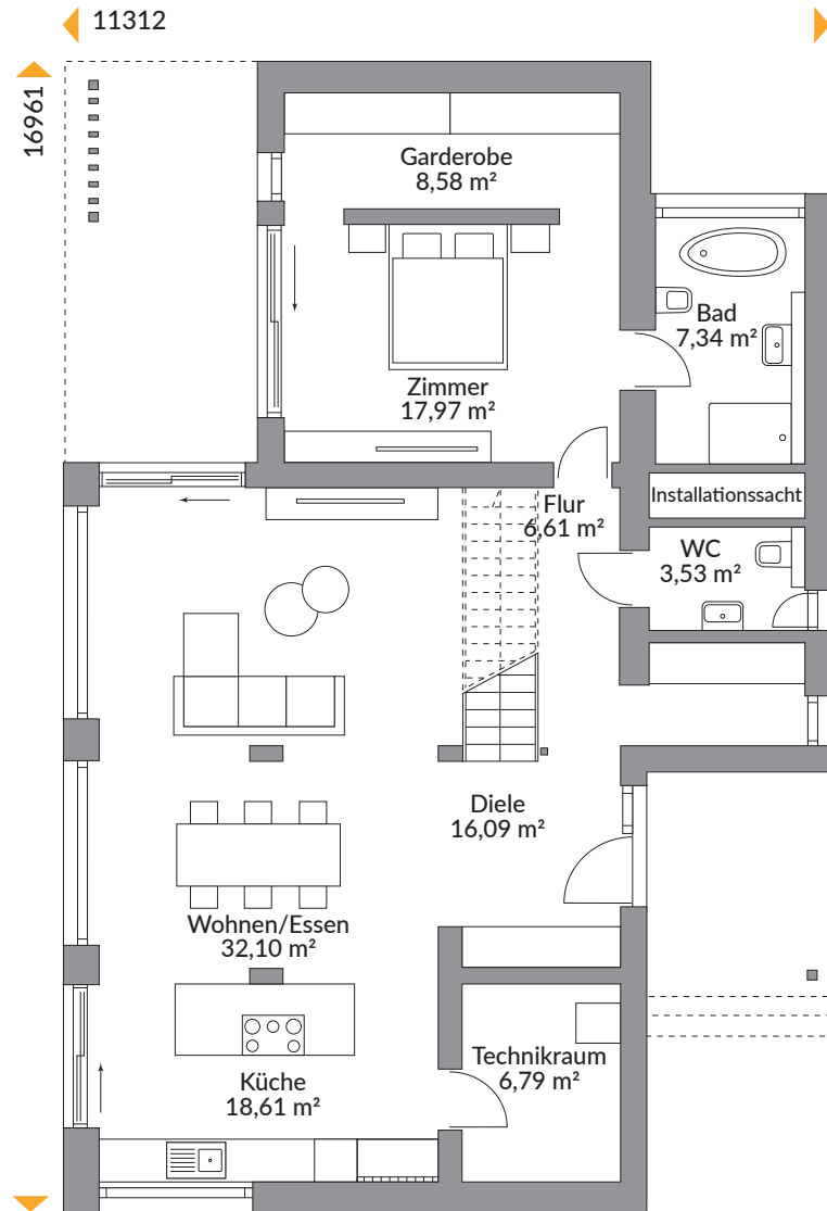
Erdgeschoss 117,62 m 2
