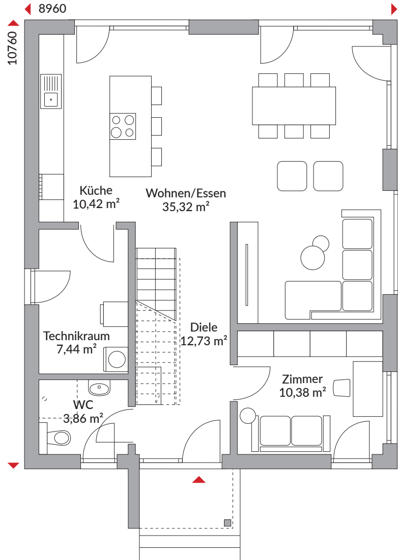
Erdgeschoss 80,15 m 2
