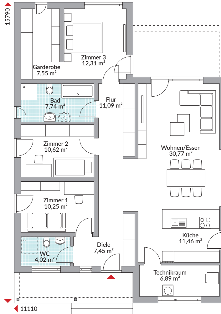
Erdgeschoss 120,15 m 2
