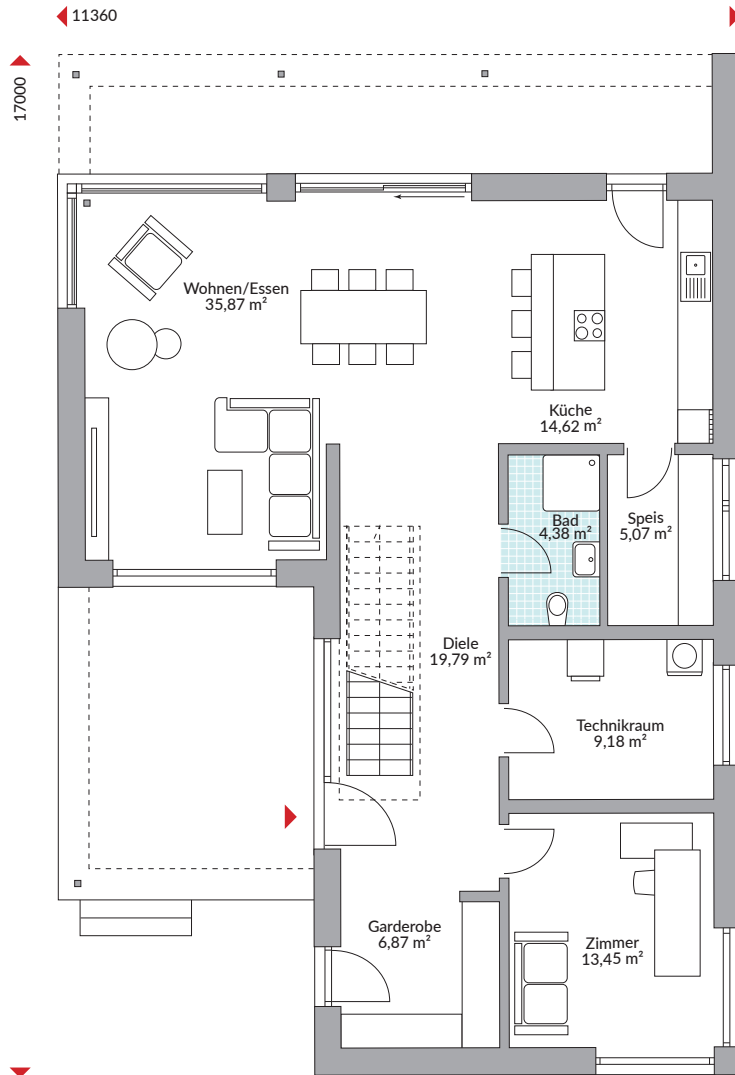
Erdgeschoss 109,23 m 2
